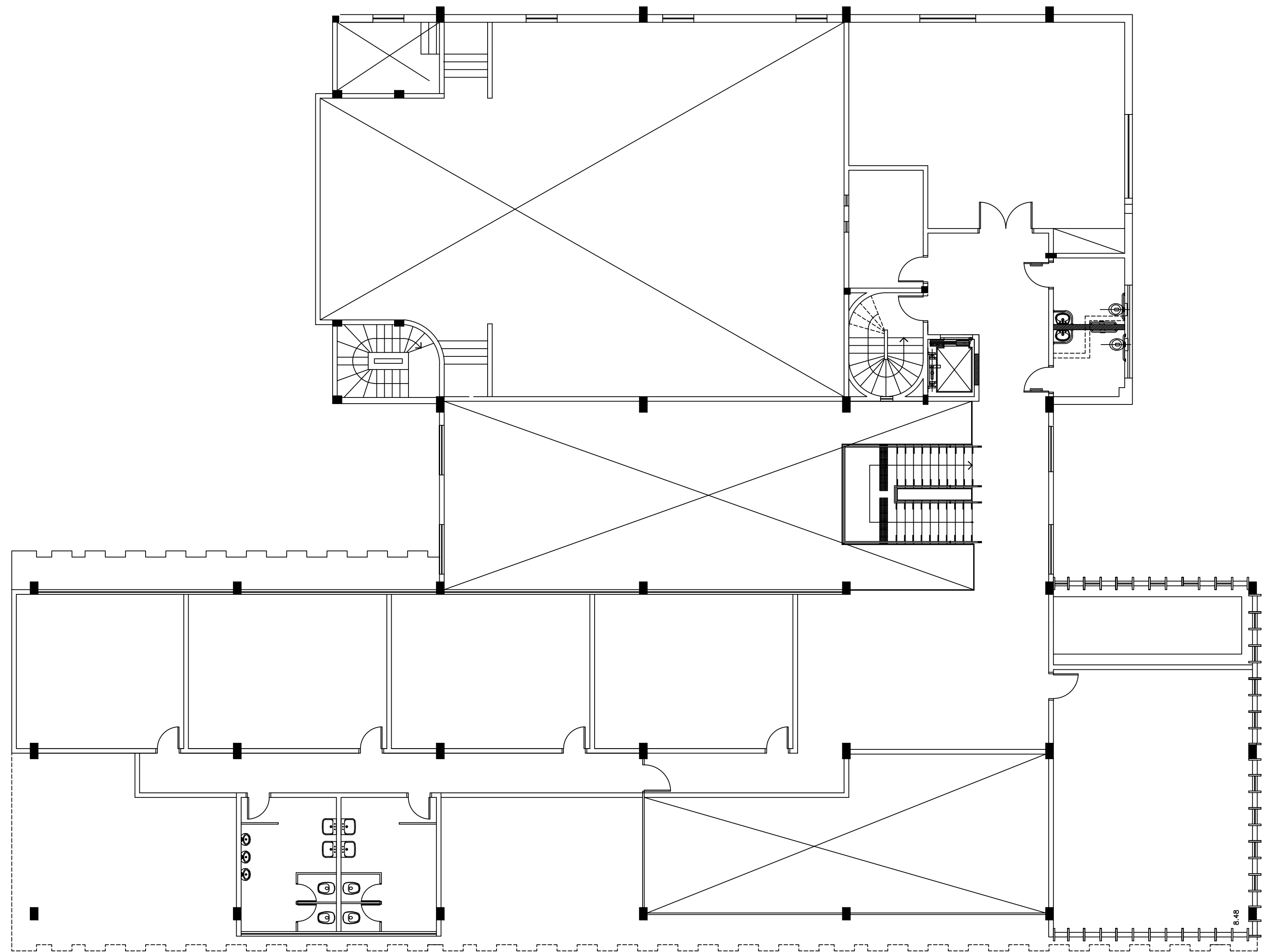
PRIMEIRO PAVIMENTO 1:100
